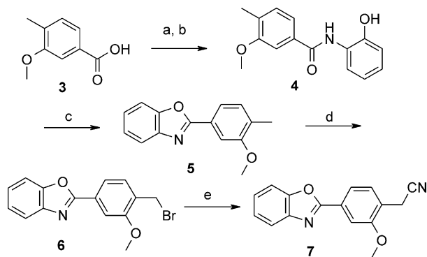
Scheme 1. Reagents: (a) SOCl 2 ; (b) 2-aminophenol, diisopropylethylamine, THF; (c) p -TsOH, toluene; (d) NBS, benzoyl peroxide, CCl 4 ; (e) NaCN, DMF.
